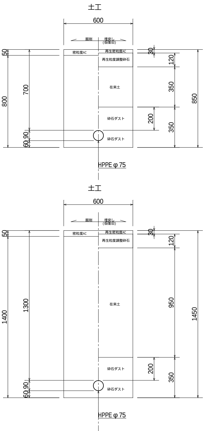
土工断面図 S=1/20
