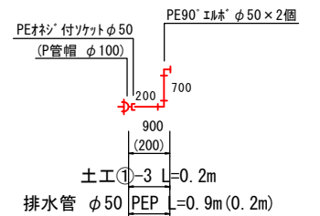
排水管詳細図(2) noscale
