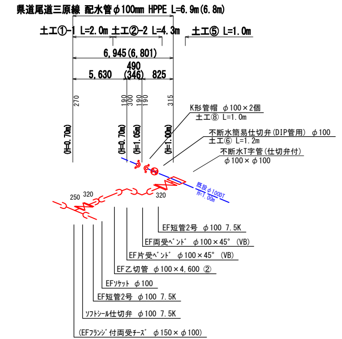
接続詳細図(2) noscale
