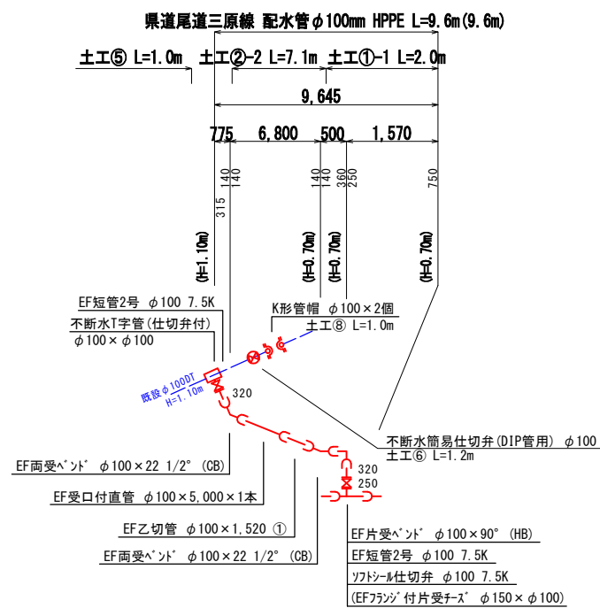
接続詳細図(1) noscale
