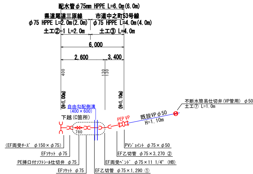
分岐工詳細図(1) noscale
