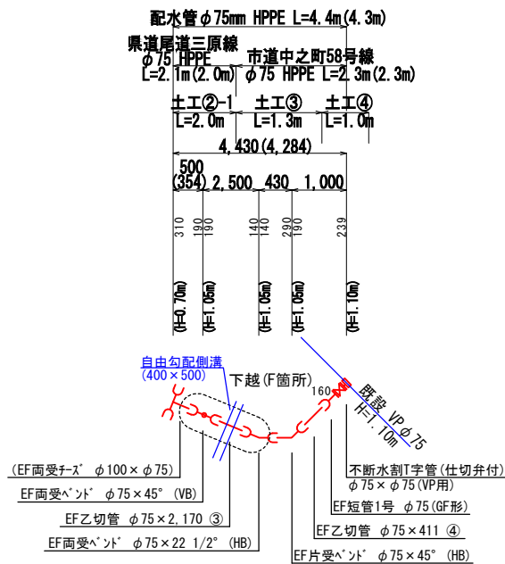
接続詳細図(3) noscale
