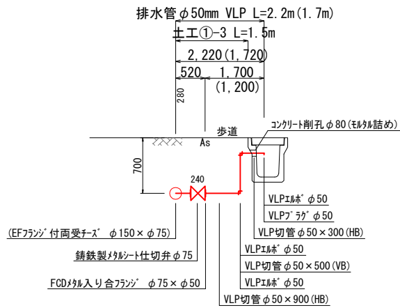
排水管詳細図(1) noscale
