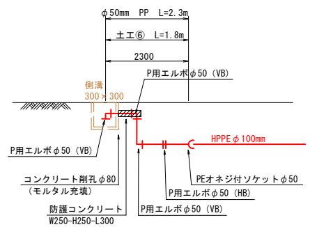
排水管詳細図
