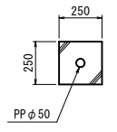
防護コンクリート S=1/20
