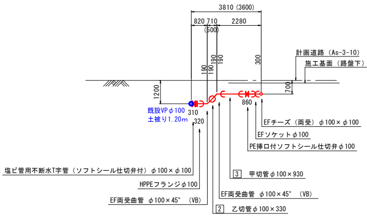
既設接続図
