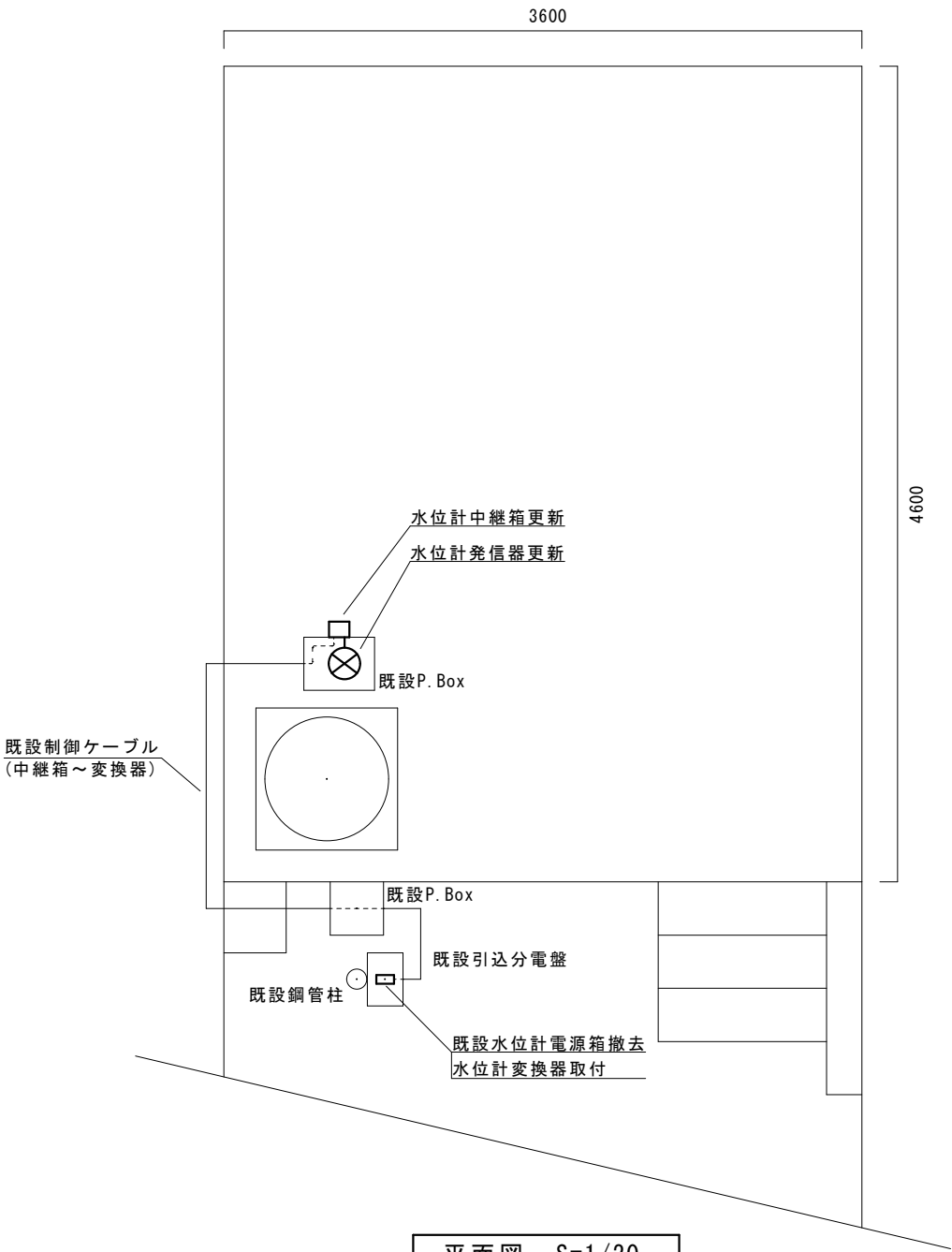
平面図 S=1/20
