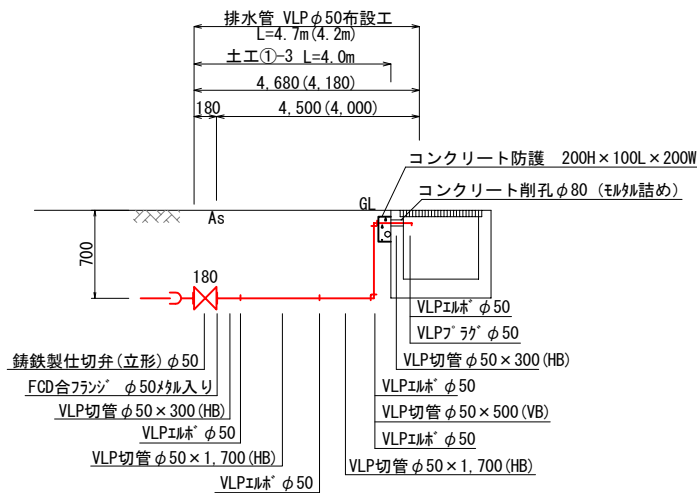
排水管詳細図1 noscale
