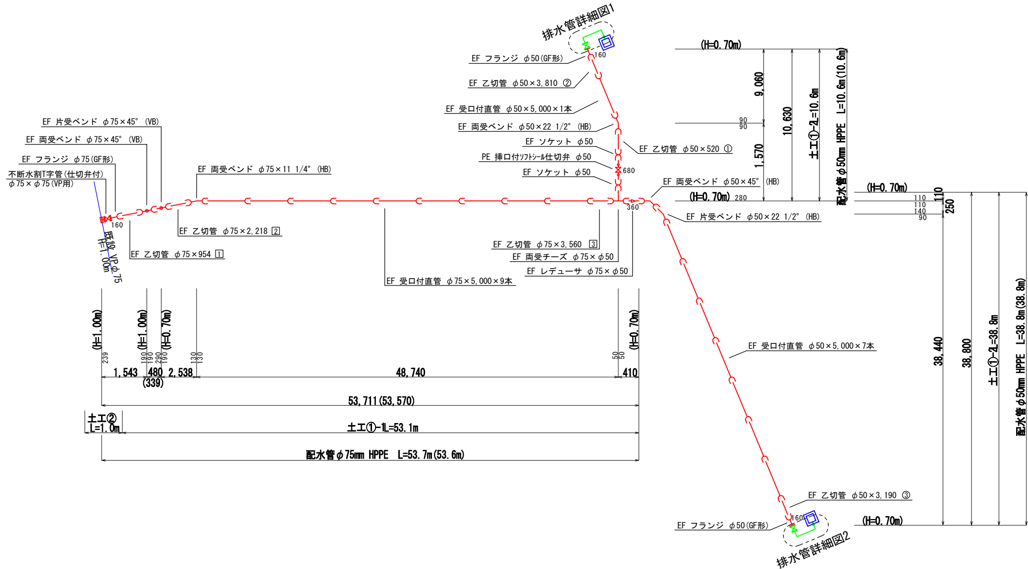
排水管詳細図1 noscale
