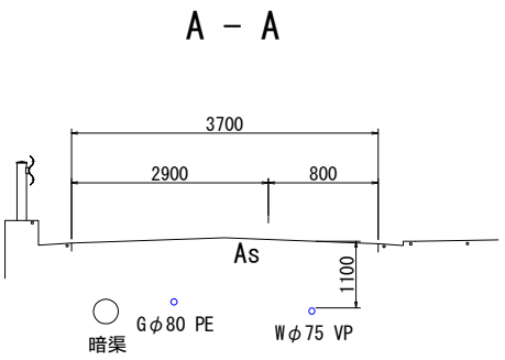
横断図 S=1:50
