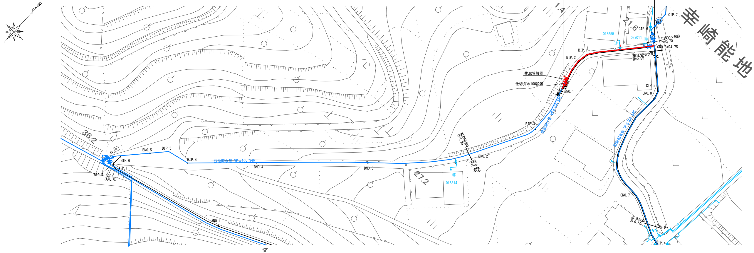
本設配水管平面図 S=1:500 (B-2路線)
