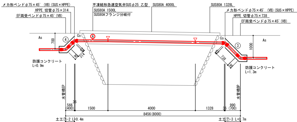
側面図 S=1:50
