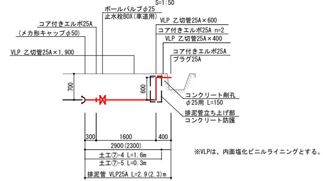
排泥管詳細図 S=1:50
