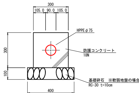
防護コンクリート詳細図 S=1:10
