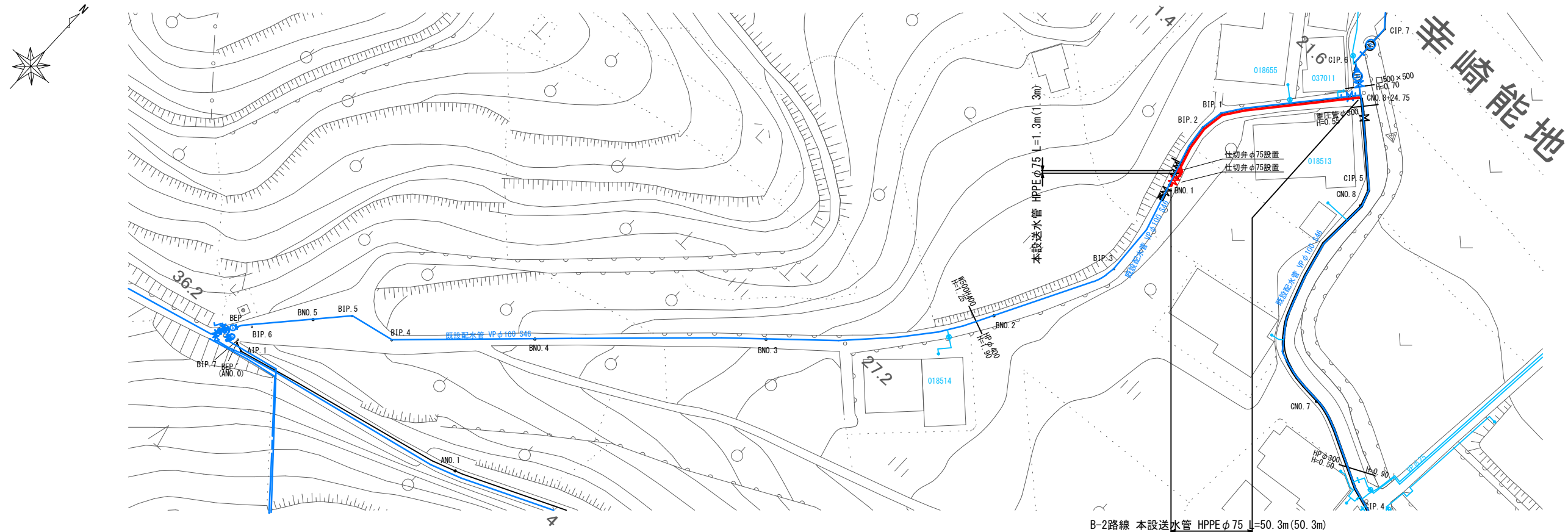
本設送水管平面図 S=1:500 (B-2路線)
