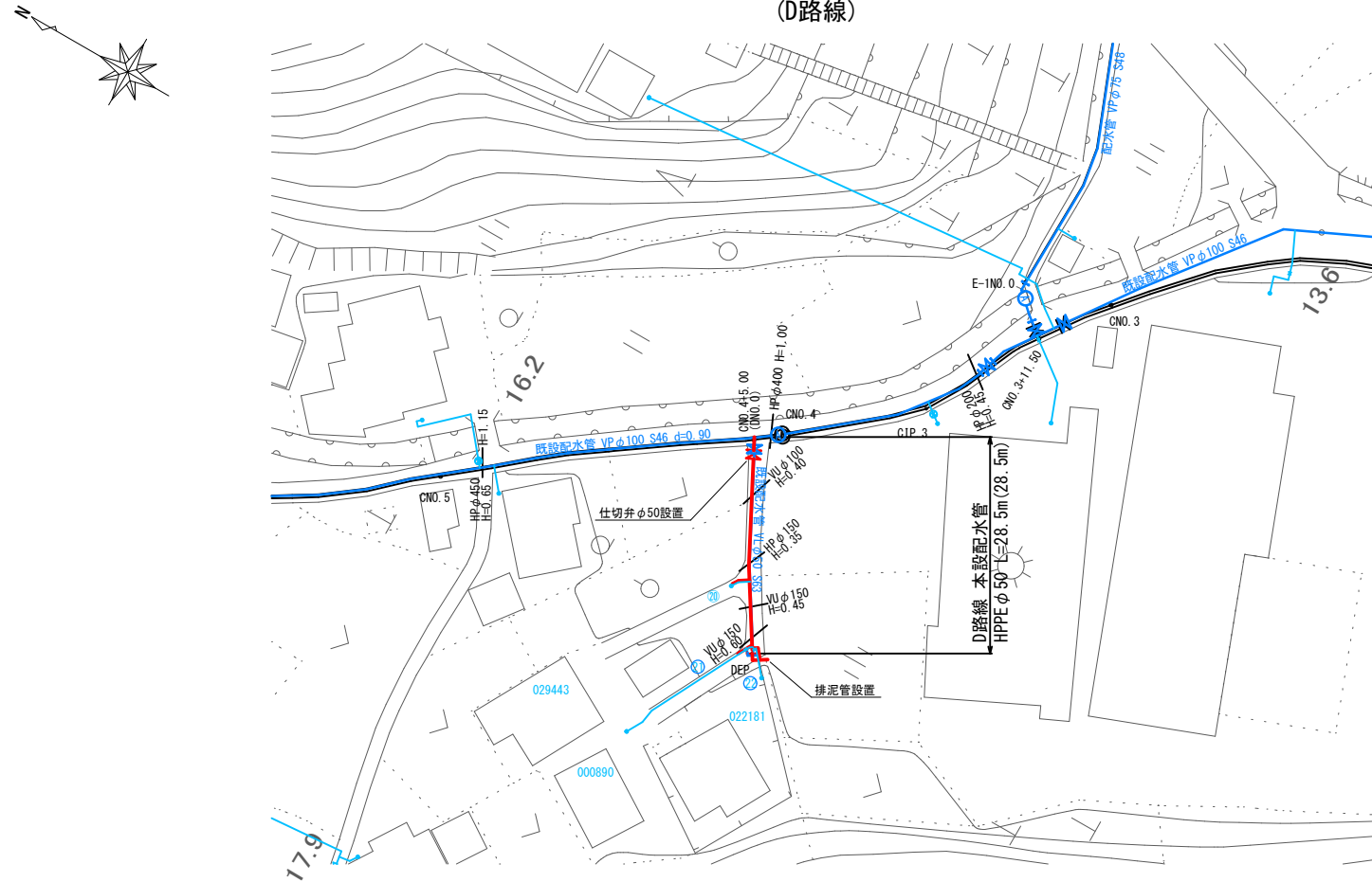
本設配水管平面図 S=1:500 (D路線)
