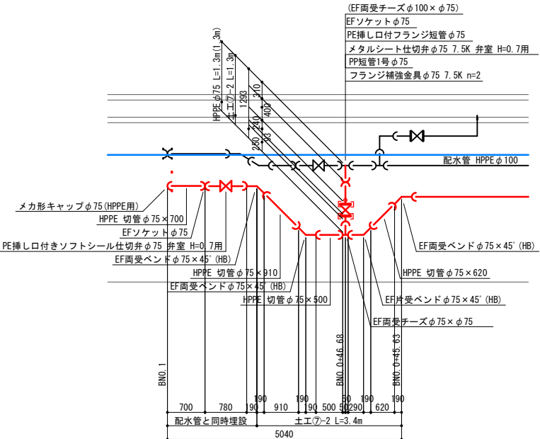
終点部詳細図 S=1:50
