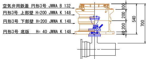
空気弁ボックス 土被りH=0.7m
