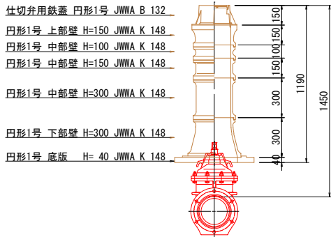
φ200仕切弁ボックス 土被りH=1.45m 不排水分岐土工1
