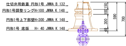
φ100仕切弁ボックス 土被りH=0.7m 不排水仕切弁土工4, 本設土工12, 13-1
