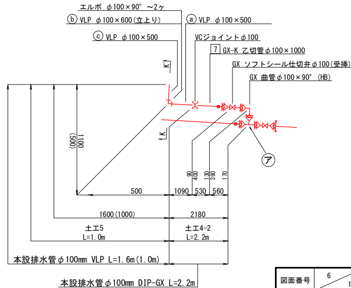
φ100排水管部詳細図 Noscale
