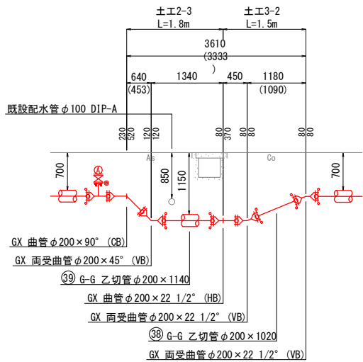
H - H' 断面図 Noscale
