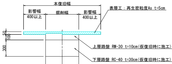
舗装本復旧図1 国道車道As
