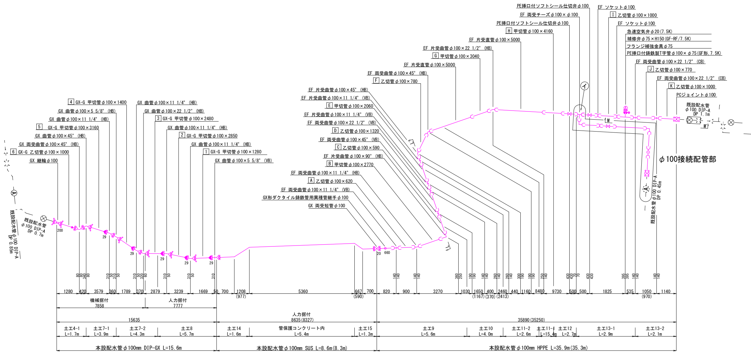
φ100接続配管部詳細図 Noscale
