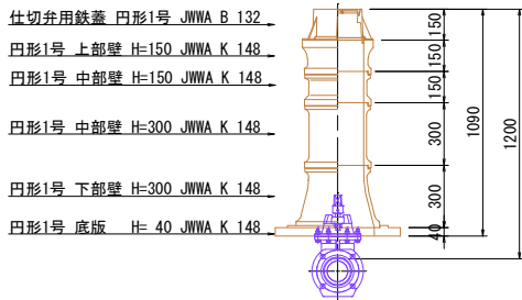
φ100仕切弁ボックス 土被りH=1.2m 不排水仕切弁土工5
