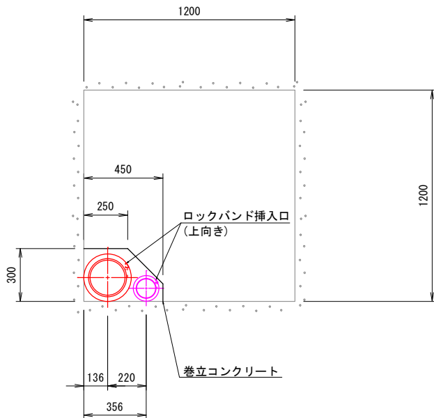
断面図 S=1/15
