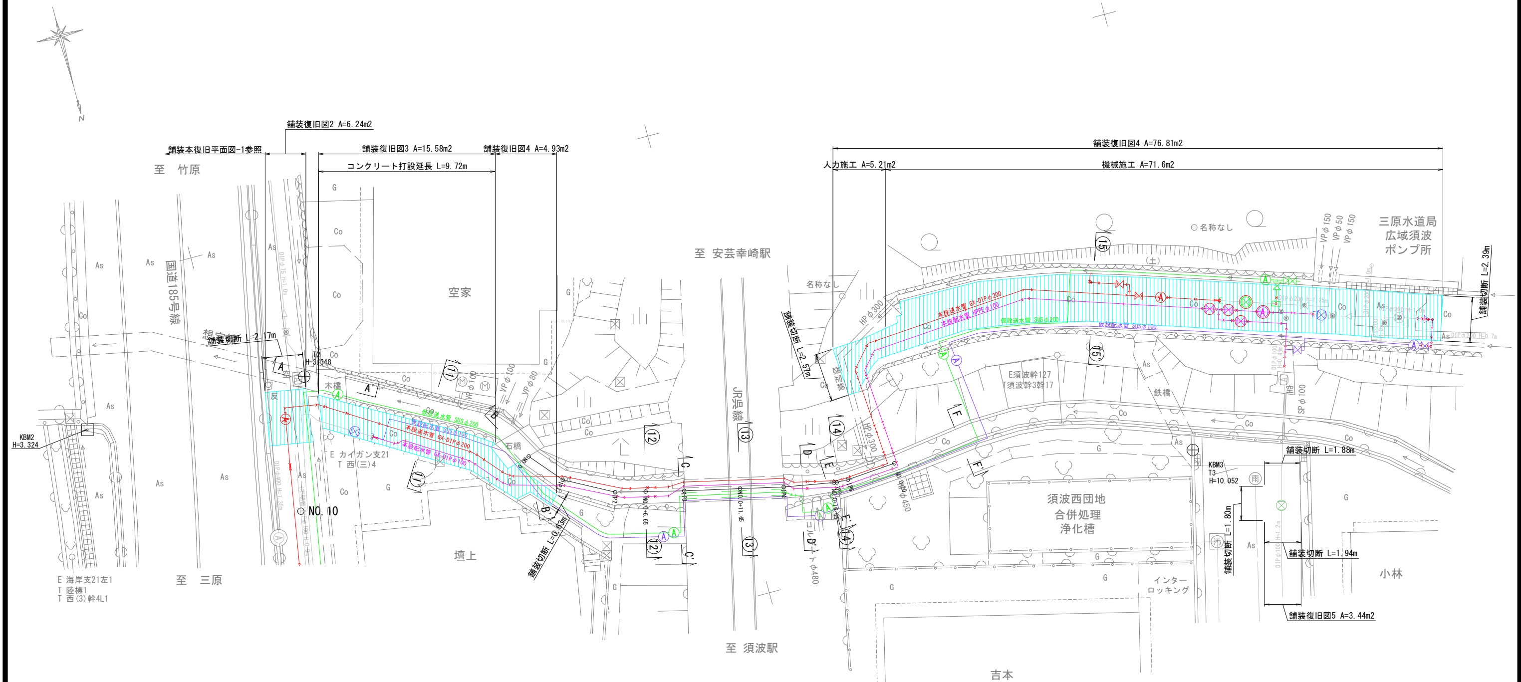
舖装本復旧図 S=1:20
