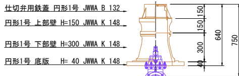
φ100仕切弁ボックス 土被りH=0.75m 本設土工4-2
