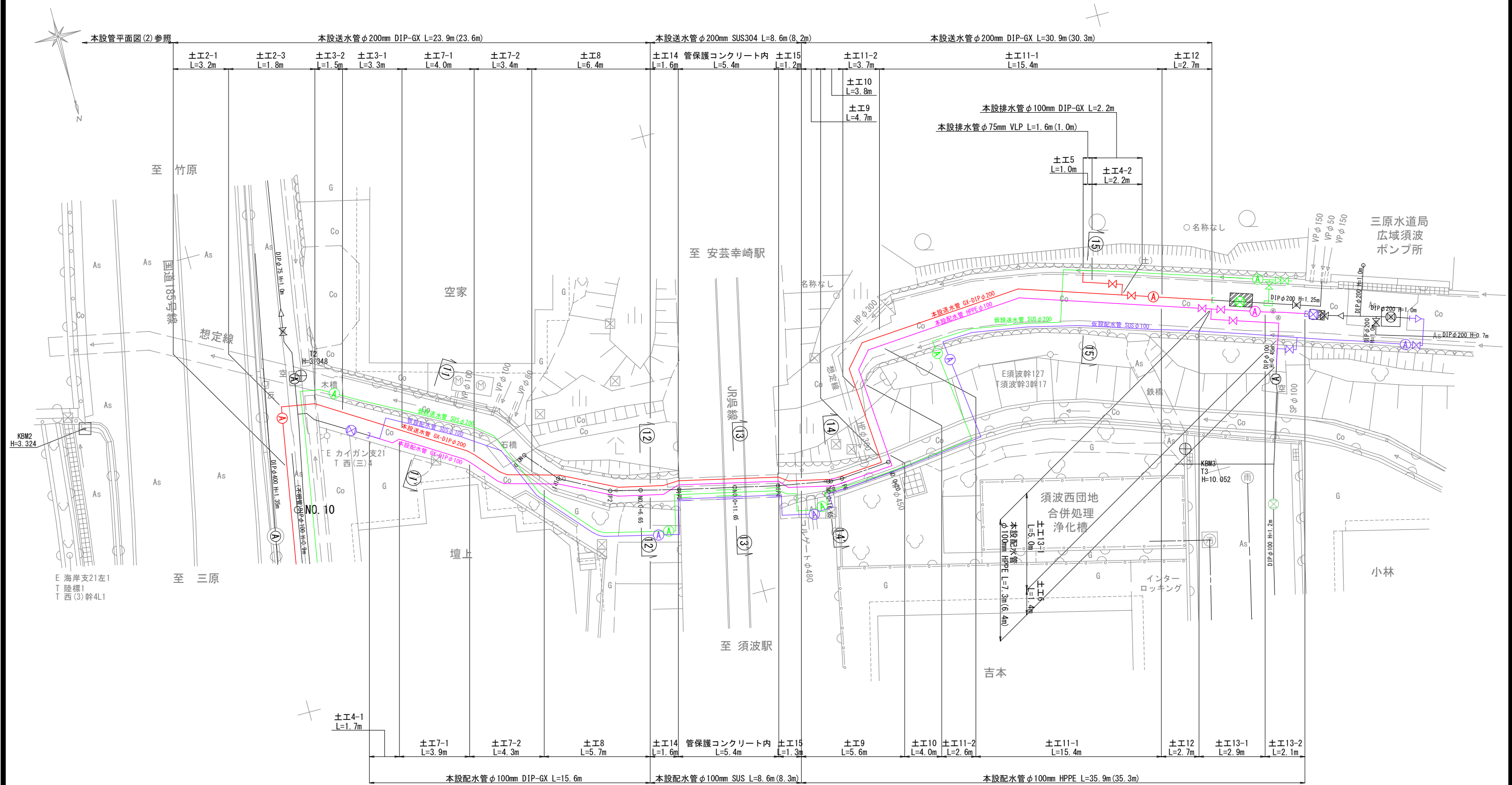
本設管平面図(3) S=1/100
