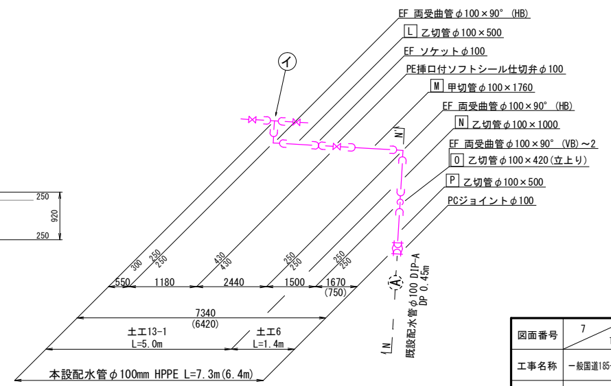
φ100接続配管部詳細図 Noscale
