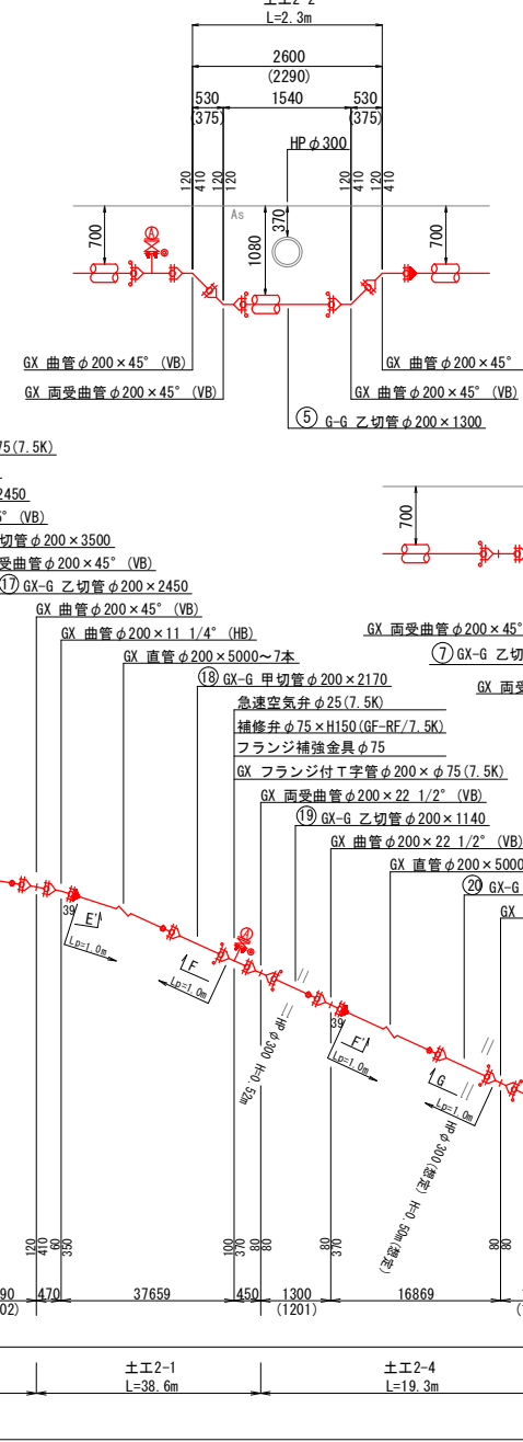
B - B' 断面図 Noscale
