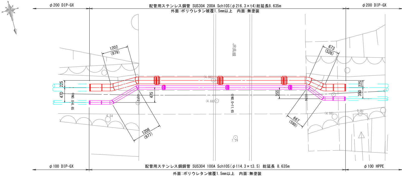
平面図 S=1/30
