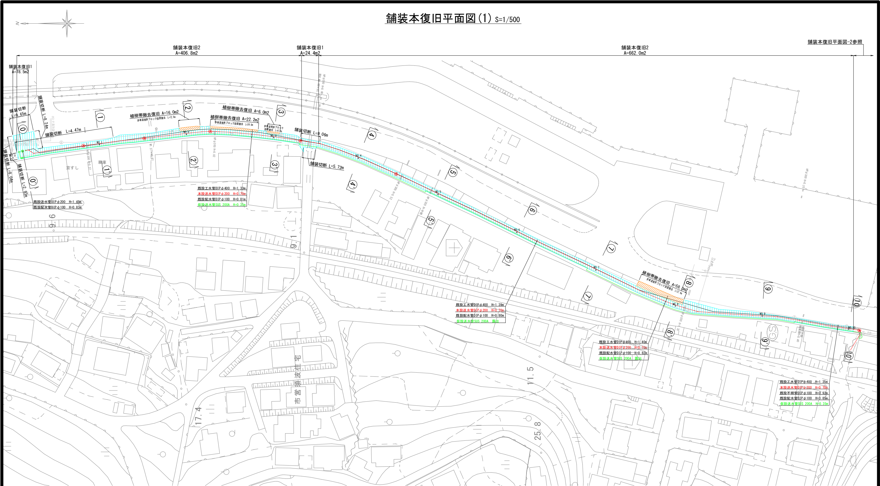
舗装本復旧図1 国道車道As
