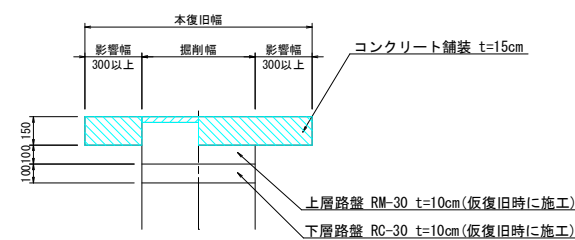
舗装本復旧図4 市道Co (JR西側)
