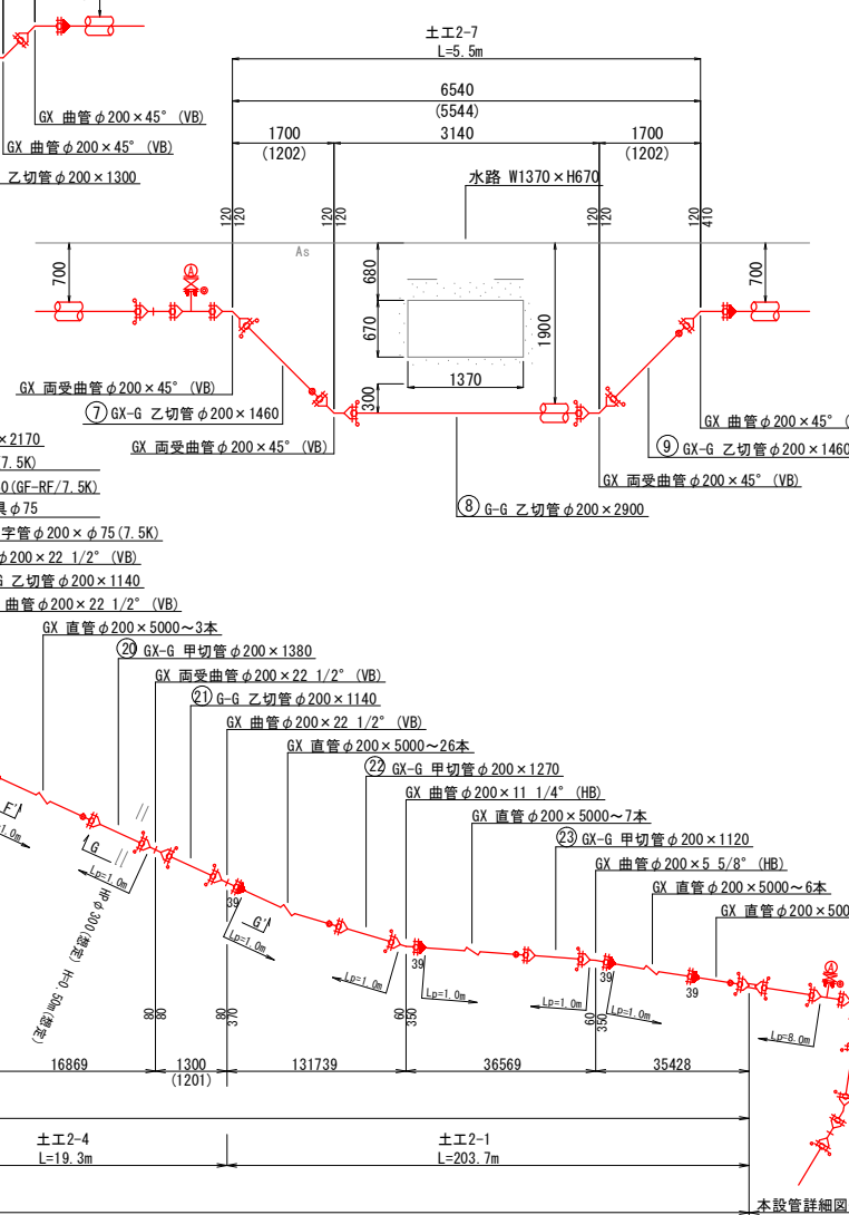
C - C' 断面図 Noscale
