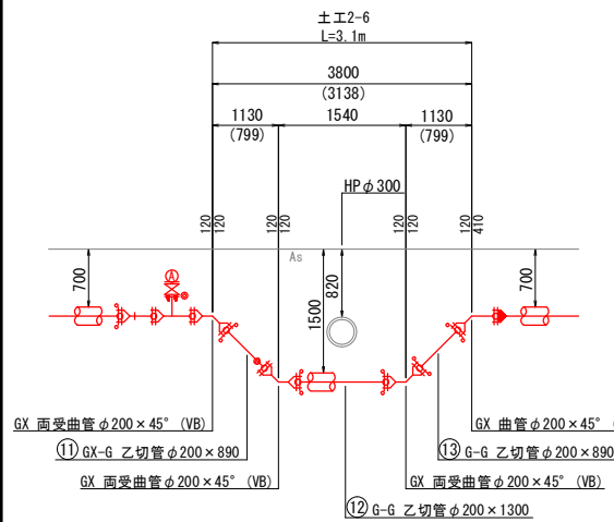
D - D' 断面図 Noscale
