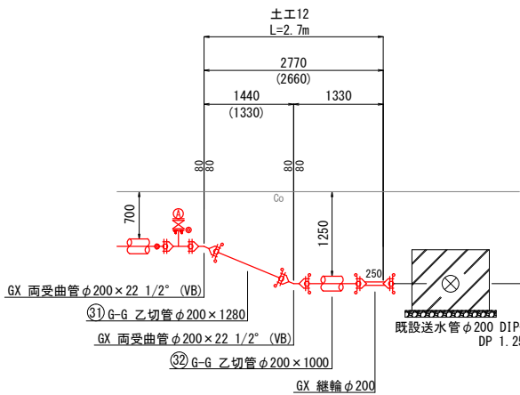
K - K' 断面図 Noscale
