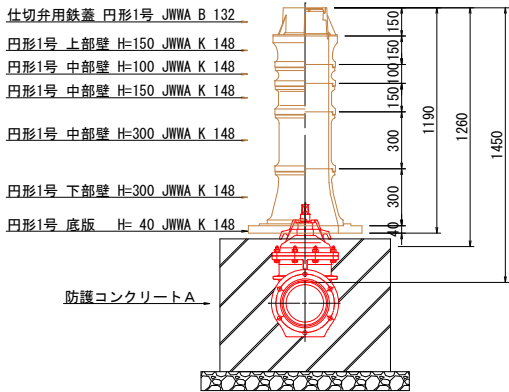
φ200仕切弁ボックス 土被りH=1.45m 不排水仕切弁土工1
