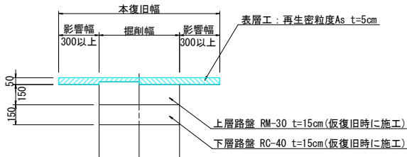
舗装本復旧図2 国道歩道As
