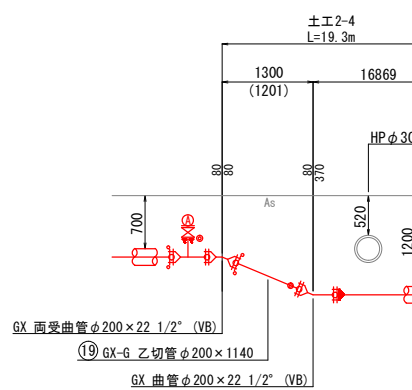
F - F' 断面図 Noscale
