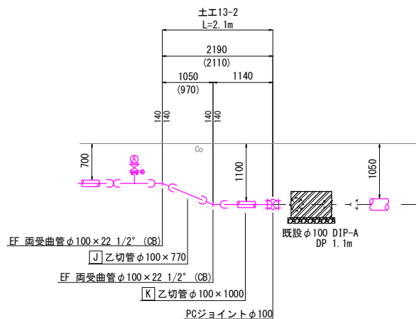
M - M' 断面図 Noscale
