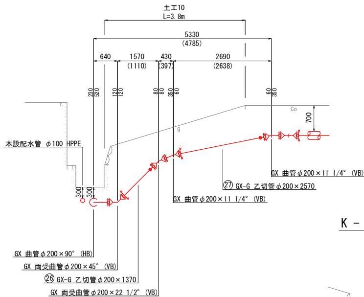
I - I' 断面図 Noscale
