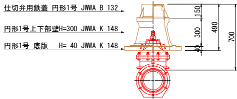
φ200仕切弁ボックス 土被りH=0.7m 本設土工11-1
