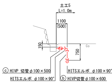
K - K' 断面図 Noscale
