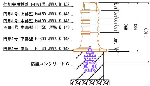
φ100仕切弁ボックス 土被りH=1.1m 不排水仕切弁土工3
