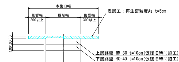
舗装本復旧図5 市道As
