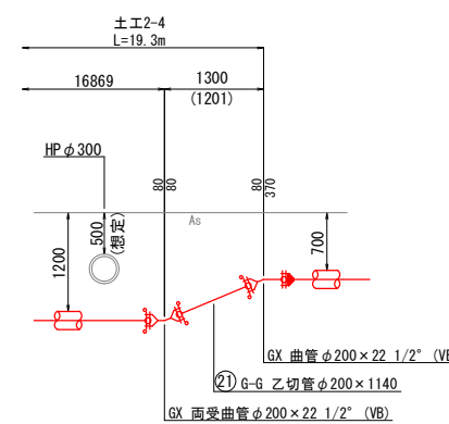
G - G' 断面図 Noscale
