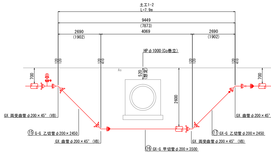
E - E' 断面図 Noscale
