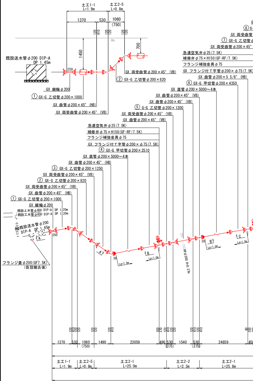
D - D' 断面図 Noscale
