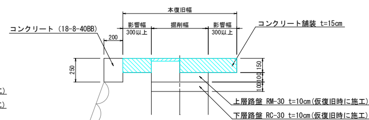
3図旧復本装舗 市道Co(JR東側)
