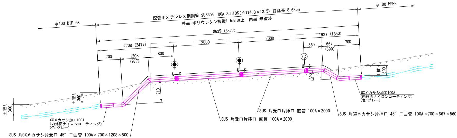
配水管 側面図 S=1/30
