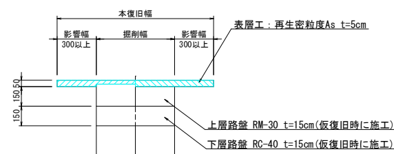
舗装本復旧図2 国道歩道As
