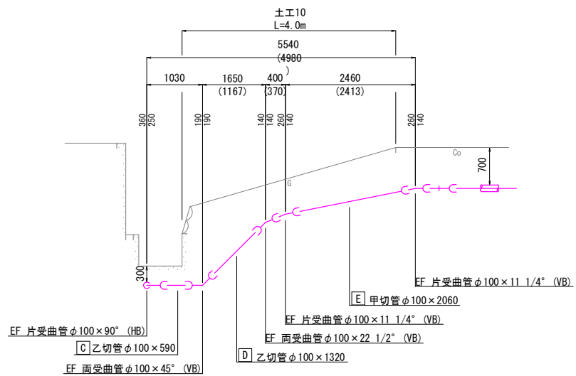
L - L' 断面図 Noscale
