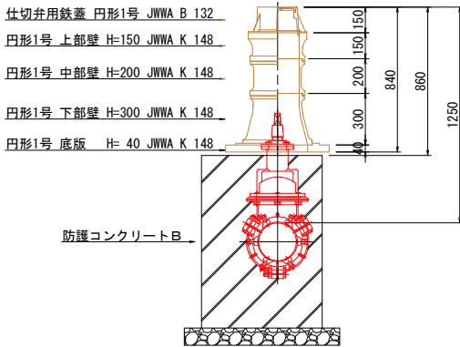
φ200仕切弁ボックス 土被りH=1.25m 不排水仕切弁土工2
