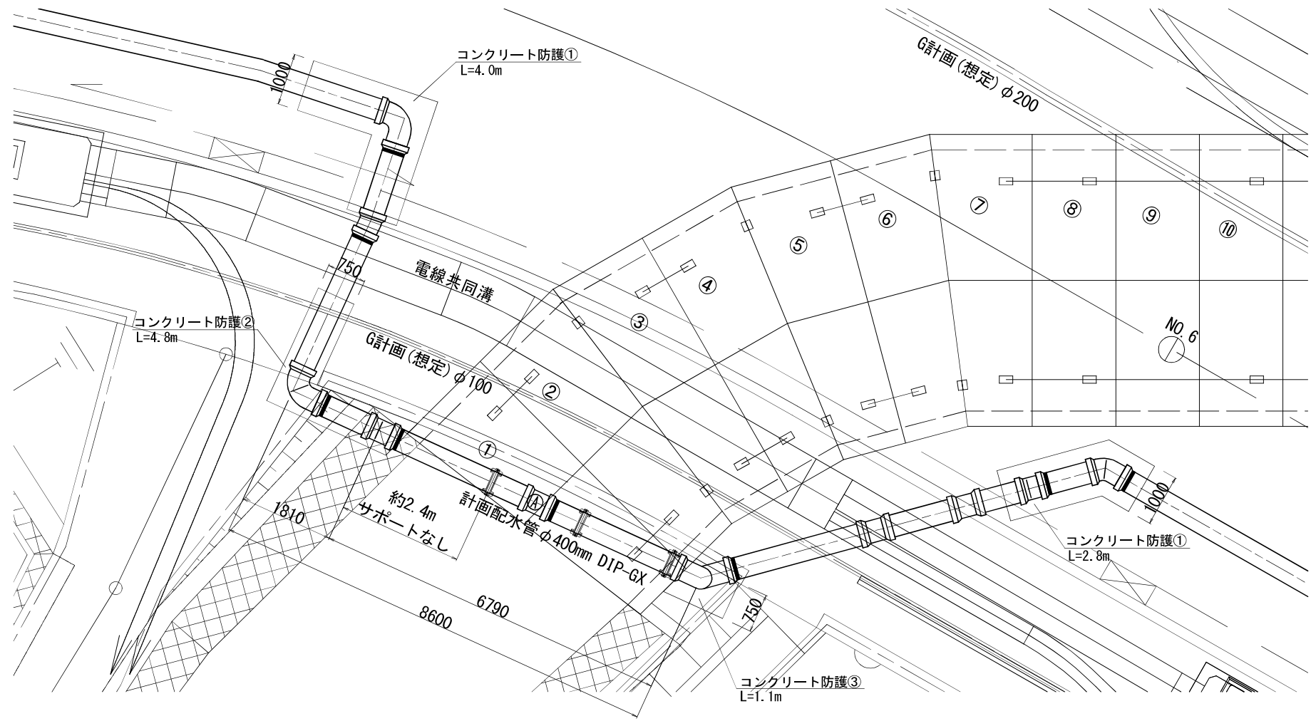
平面図 S=1:50
