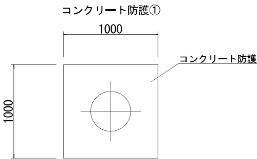
コンクリート防護詳細図 S=1:20
