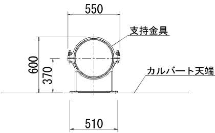
断面図 S=1:20
