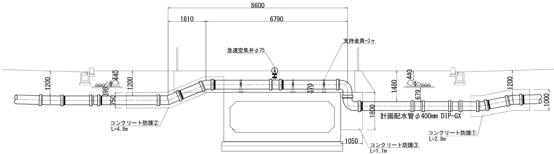
縦断面図 S=1:50
