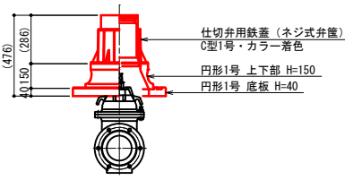
仕切弁 φ150 H=0.60m 不斷水仕切弁 φ150 H=0.60m
