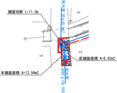
As舗装部 舗装復旧平面図 S=1:250
