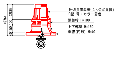
仕切弁 φ75 H=0.60m
