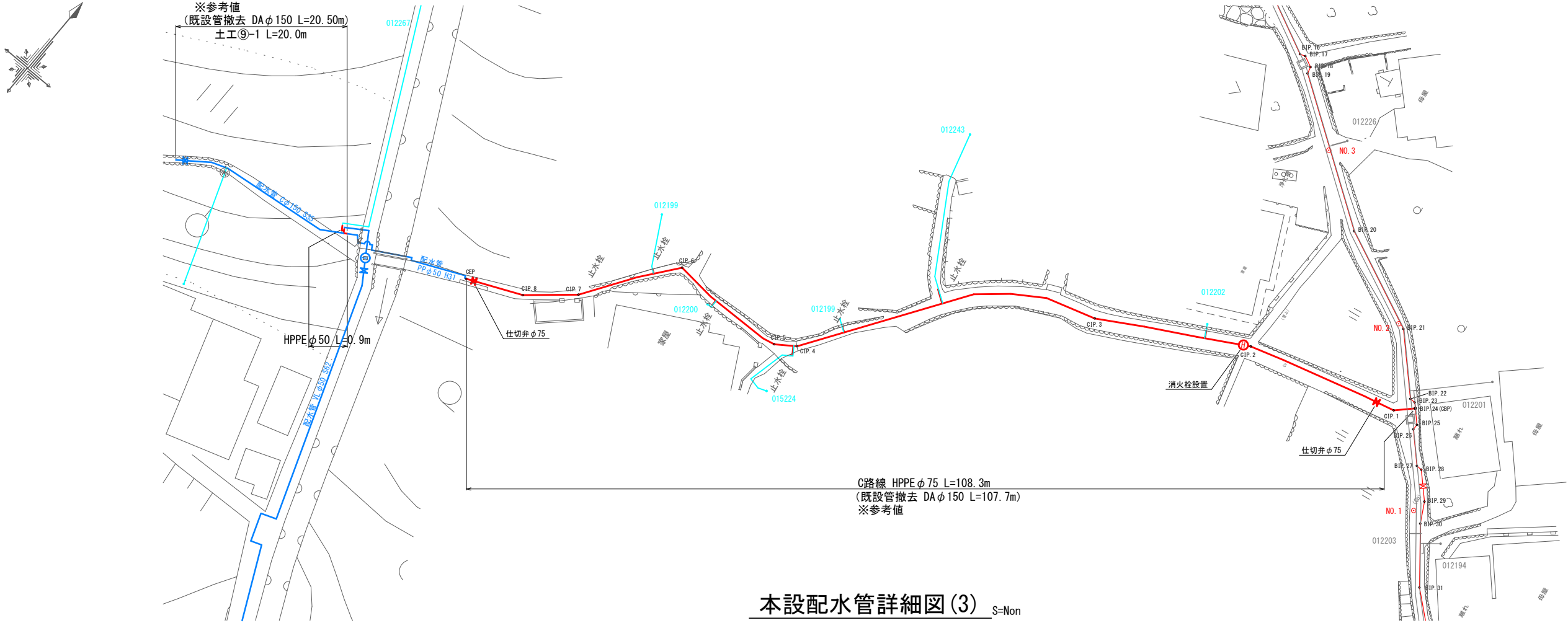
本設配水管平面図(3) S=1:250
