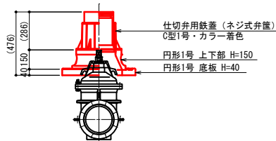
仕切弁 φ200 H=0.60m
