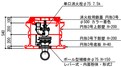
消火栓 φ75 H=0.60m
