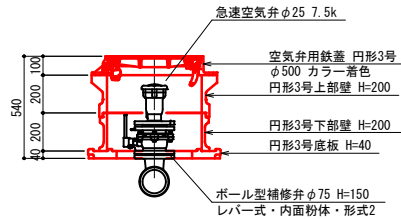
空気弁 φ25 H=0.60m
