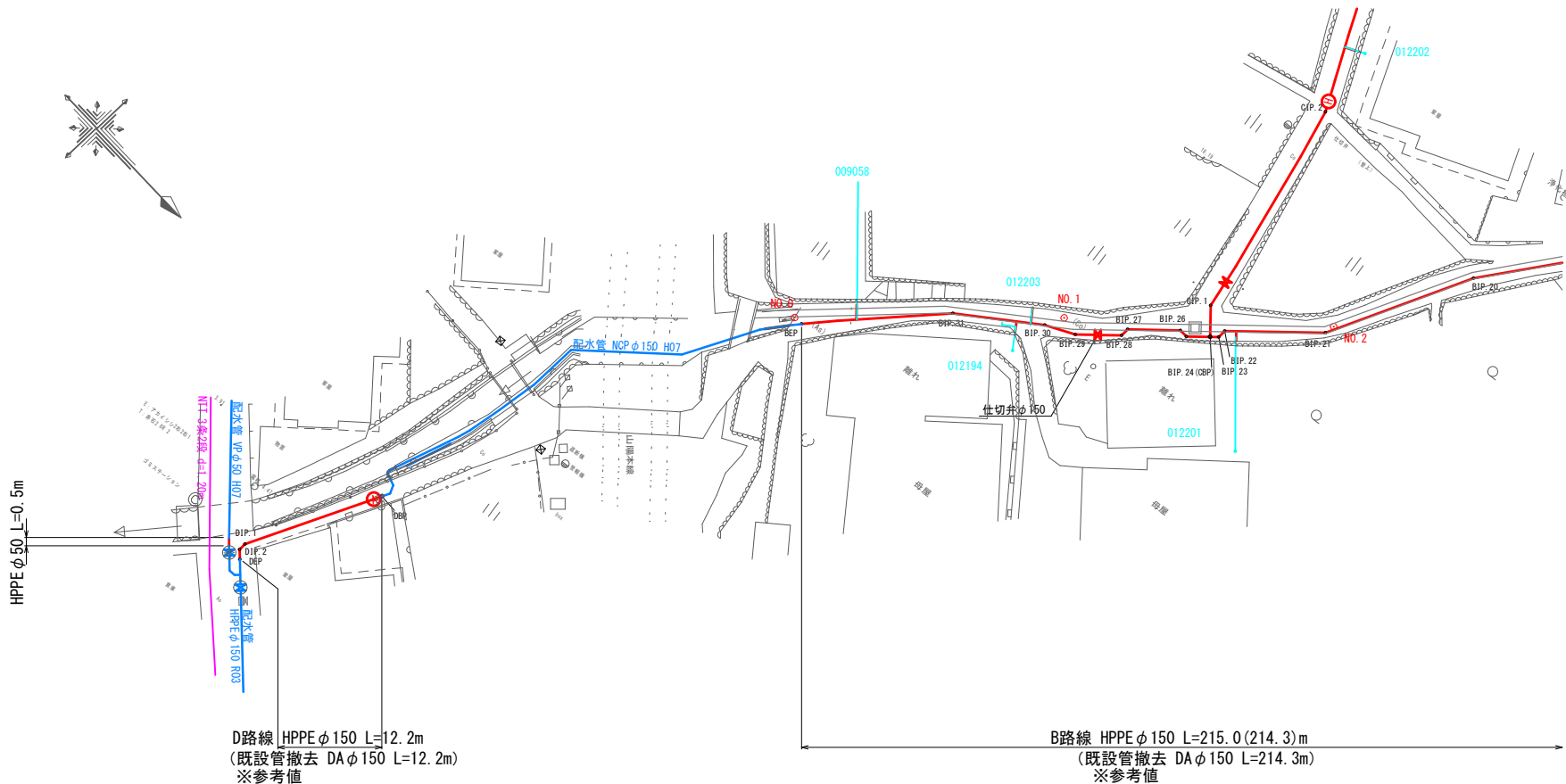
本設配水管平面図(2) S=1:250
