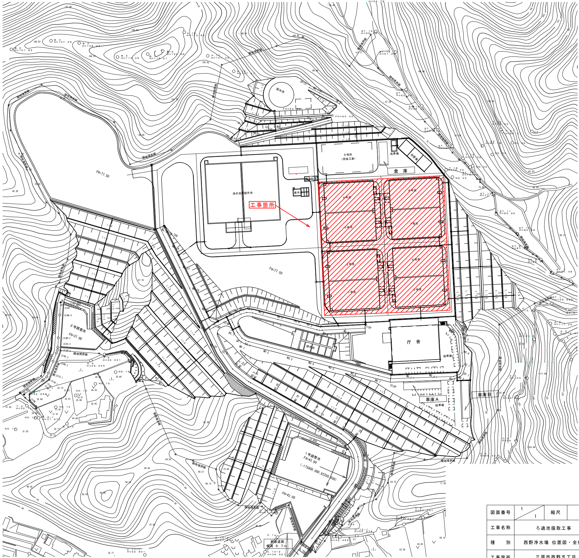
西野浄水場全体平面図 (S=1/1000)
