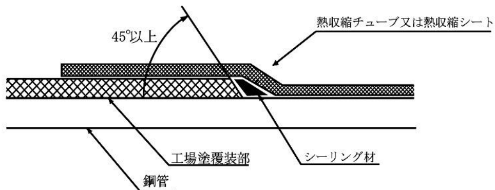
図 15-1-6 シーリング材の施工
