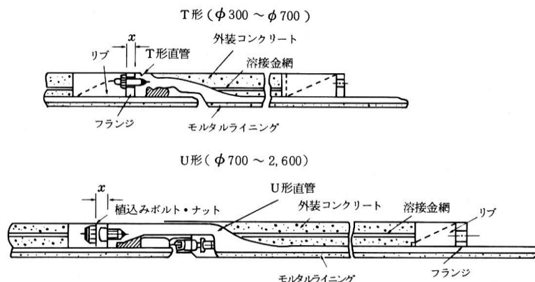
図 15-1-6 推進工法用ダクトイル管の構造
