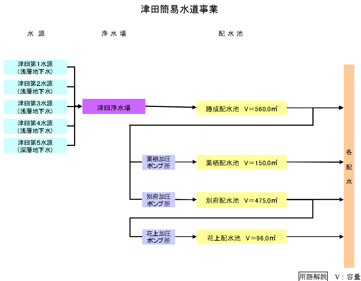
図 9 配水フロー（津田簡易水道事業）
