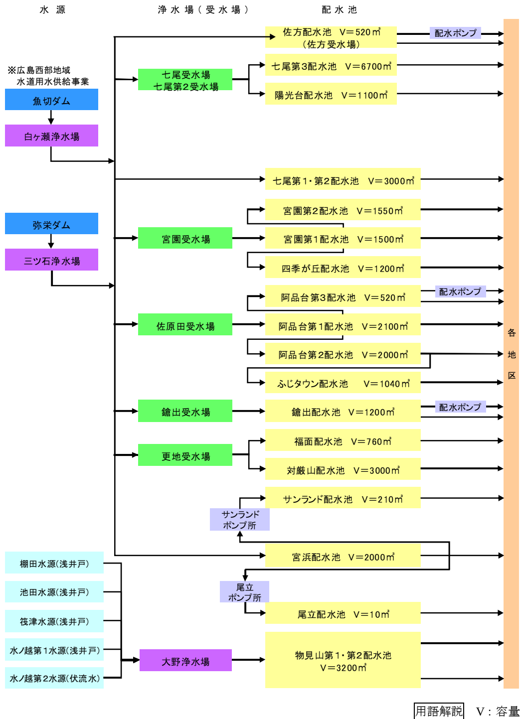
図 3 配水フロー（上水道 廿日市地域及び大野地域）
